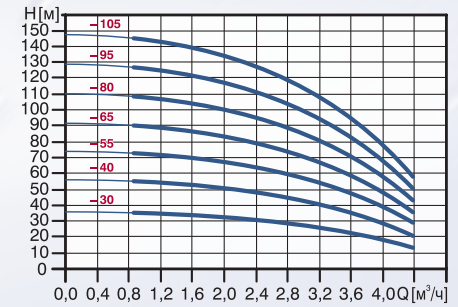
SQ 3 / SQE 3
