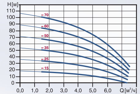
SQ 5 / SQE 5
