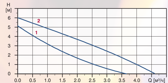
SOLAR 25-60
