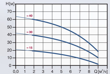
SQ 7 / SQE 7
